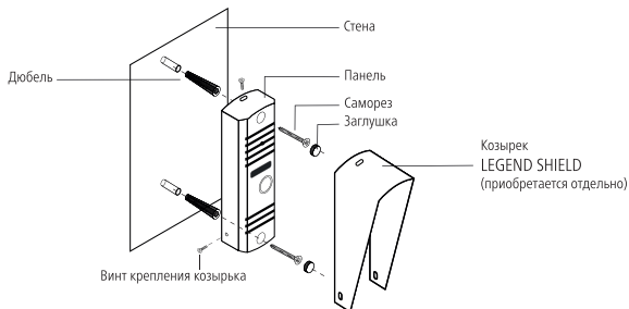
Рис. 8 Фронтальная установка вызывной панели
