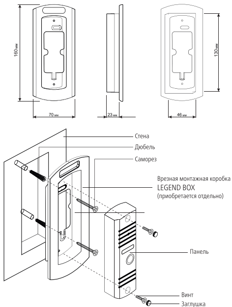
Рис. 10 Врезной монтаж вызывной панели
