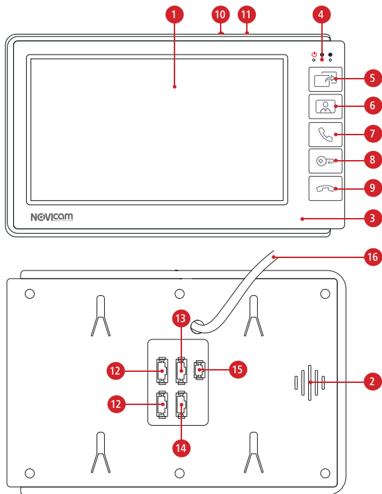
Рис. 3 Описание монитора SMILE 7 HD
