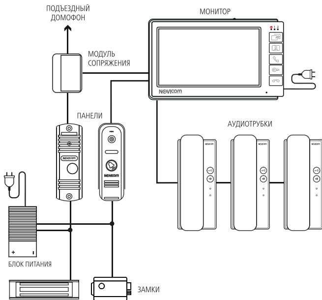
Рис. 11 Функциональная схема системы на базе видеодомофона SMILE 7 HD
