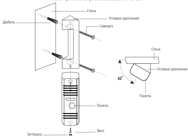
Рис. 9 Установка вызывной панели под углом 30°
