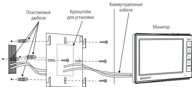
Рис. 7 Монтаж монитора
