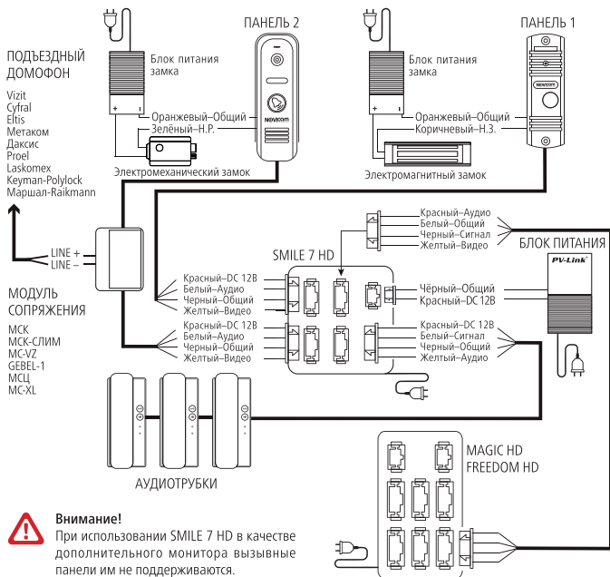
Рис. 12 Схема подключения видеодомофона SMILE 7 HD
