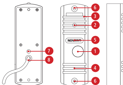
Рис. 2 Описание вызывной панели LEGEND HD
