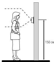
Рис. 3 Рекомендуемая высота установки видеопанели
